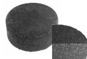
links: Bohrkern-Verschluss, Ø 15 cm, rechts: im Anschnitt Bite auch hier in Lagen einbauen und verdichten
